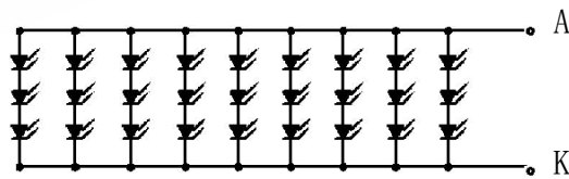
LED 电路图
